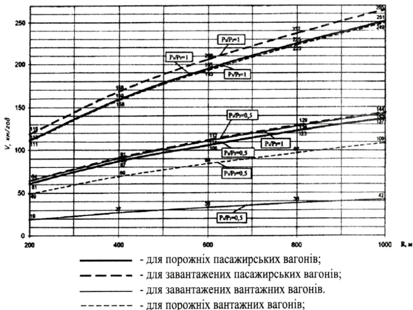
Рис. 3. Графіки залежності допустимої швидкості руху стрілочними переводами за умови недопущення наповзання колеса на рейку при нормативному значенні коефіцієнта стійкості K_{уст}^{нап} = 1,5
