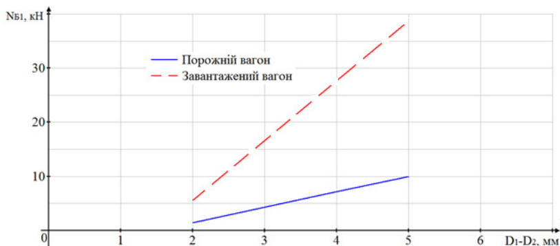
Рис. 3. Залежність сили N_{B1} від різниці діаметрів коліс D_1 - D_2
