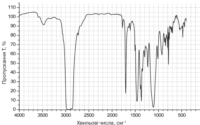
Рис. 4. ІЧ-спектр поглинання товарного зразка присадки Octimise G2003, шар товщиною 0,024 см.
