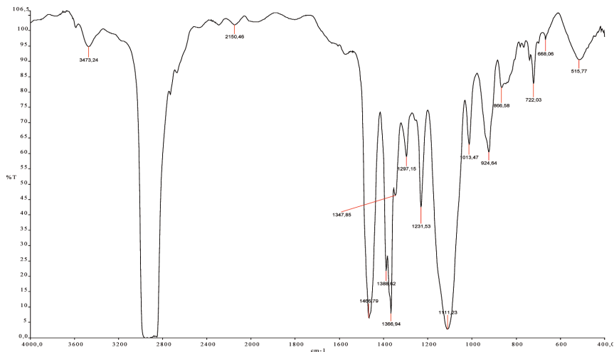
Рис. 2. ІЧ-спектр поглинання присадки «Keropur R Pulsar 2» виробництва концерну BASF, THK, шар товщиною 0,024\text{ см} .
