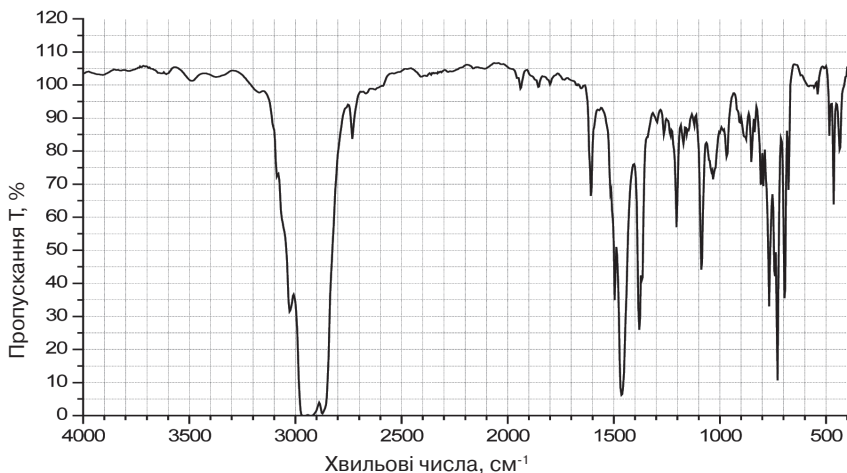
Рис. 5. ІЧ-спектр поглинання бензину марки АИ-92 Євро.
