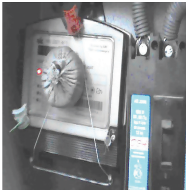
Рис. 2. Електронно-механічний лічильник із встановленим на ньому магнітом для безоблікового споживання електроенергії
