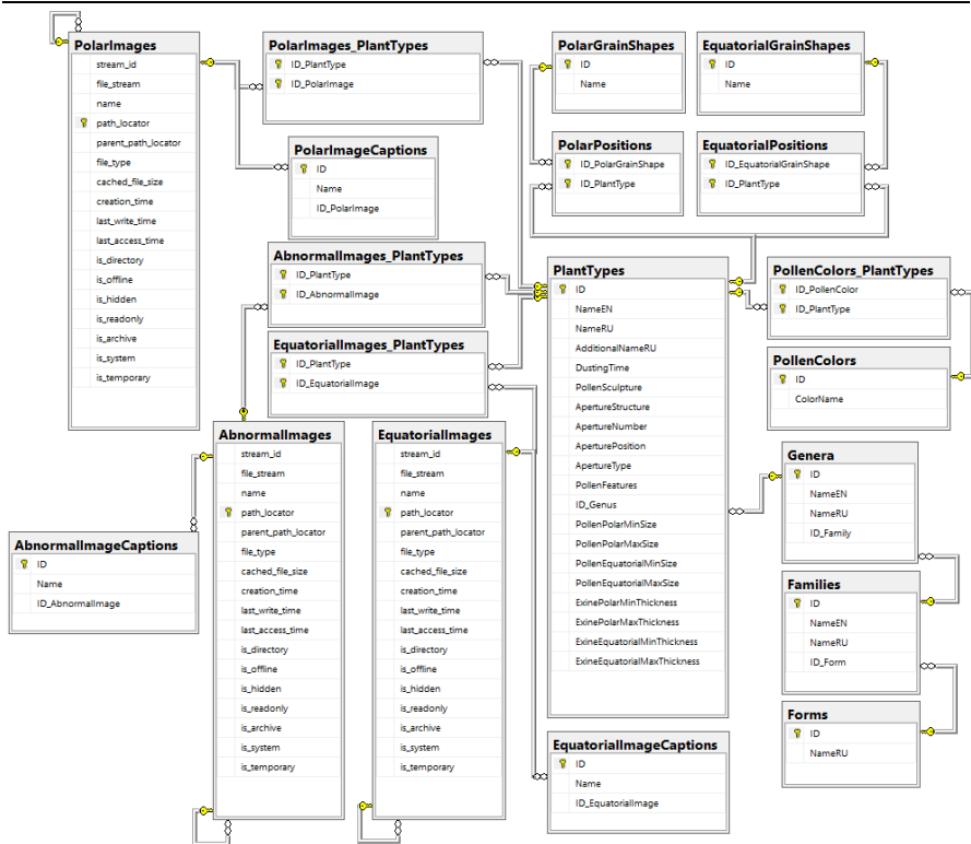
Рис. 3. Структура СИПС «PalExp»
